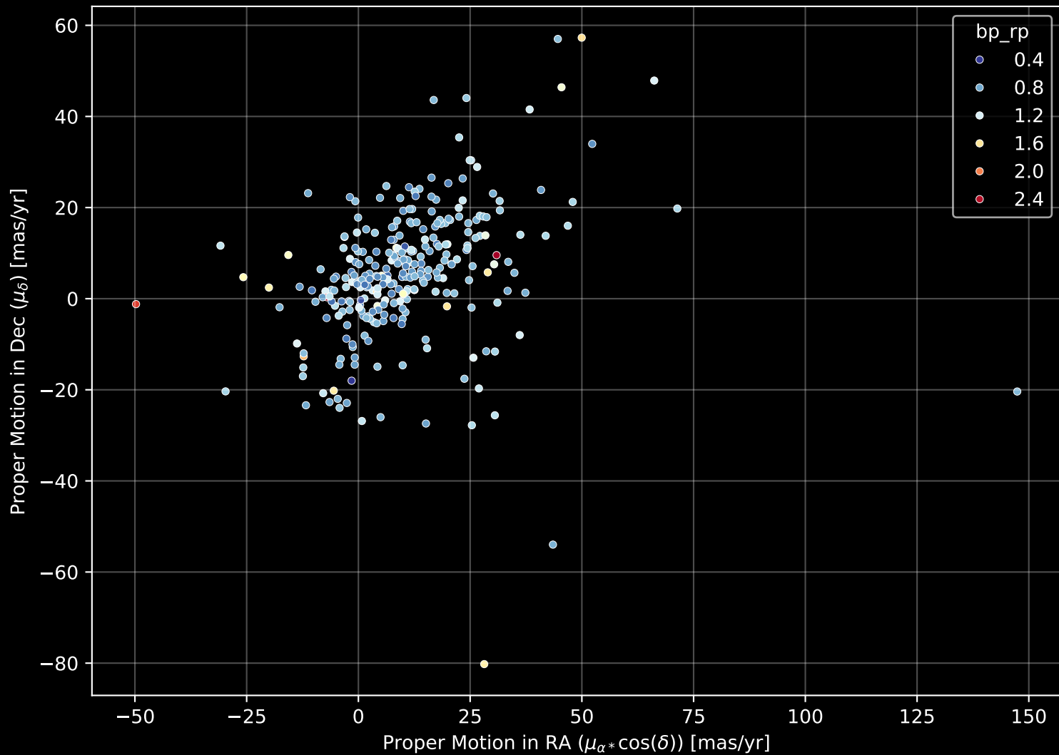
GALAH DR4 Field: [180] Proper Motion Diagram (n= 294)
