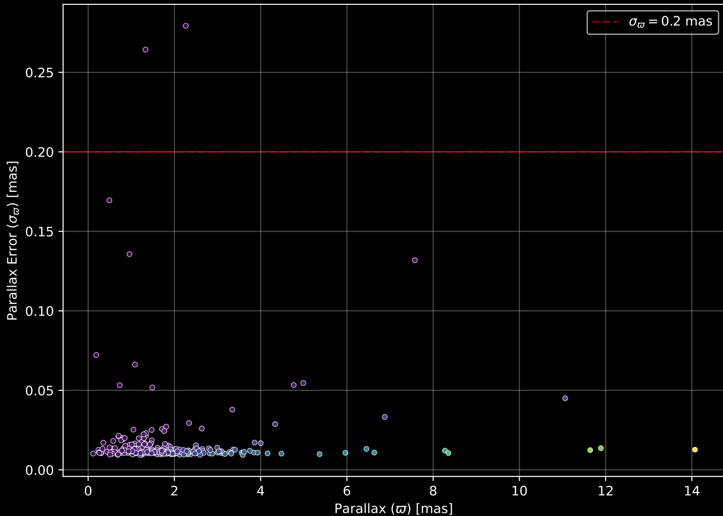
GALAH DR4 Field: [180] Parallax Quality (n= 294)
