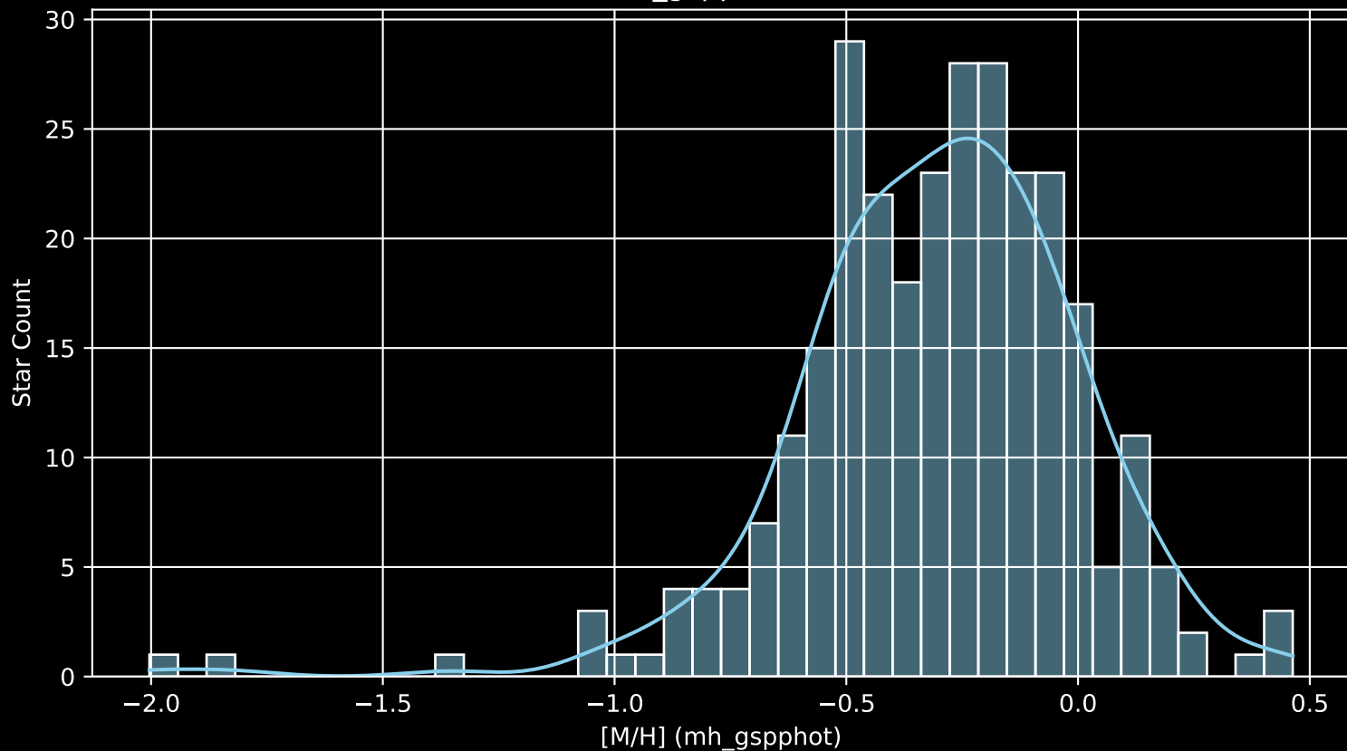
GALAH DR4 Field: [180] [M/H] (mh_gspphot) (n= 291)
