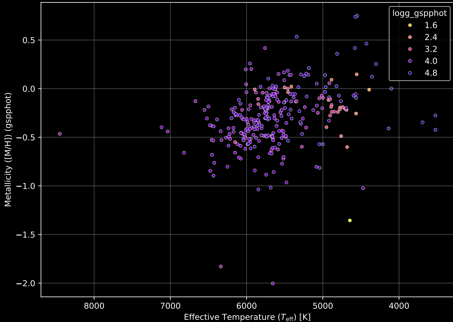
GALAH DR4 Field: [180] Stellar Population Parameters (n= 294)
