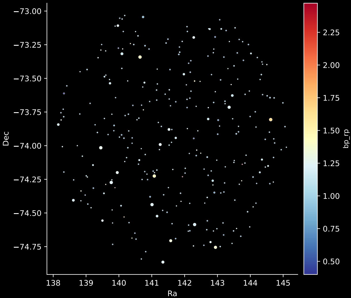
GALAH DR4 Field: [180] Stars: 294
